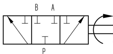
O型原理图
