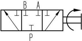
0型原理图
