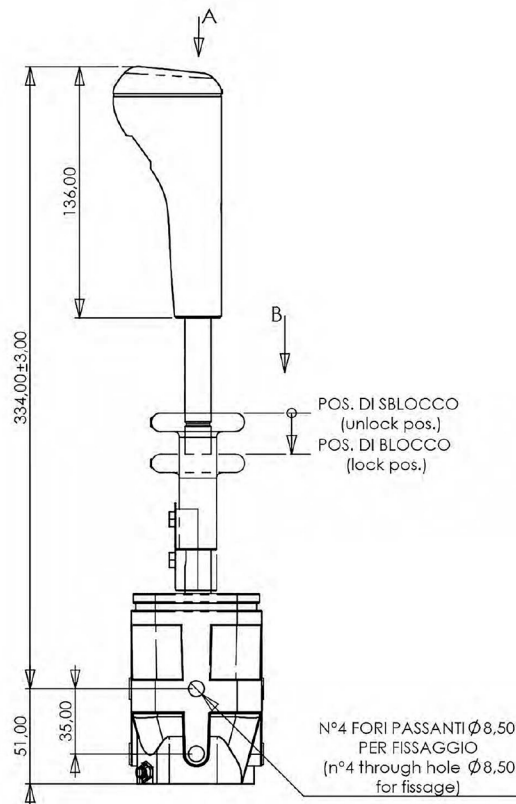
VISTA PARZIALE (partial view)
